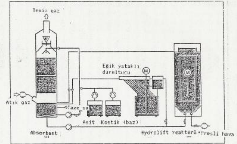
Sekil 5 : Bir biyokatalitik atıkgaz arıtma tesisinin yavaş işleme akışının şeması
