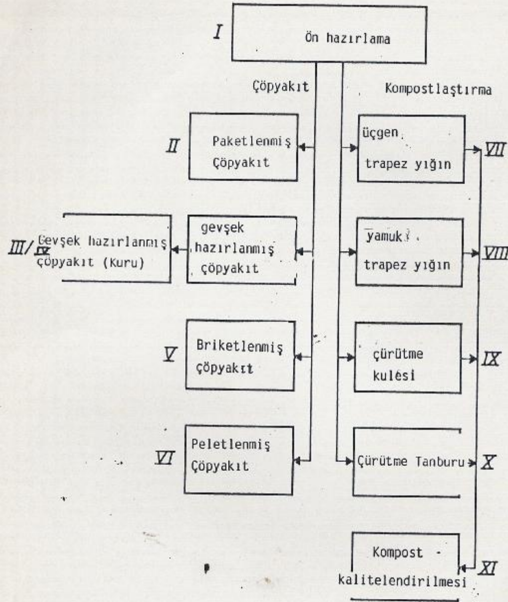
Şekil : Çöpten kompost ve çöpyakıt eldesi için yöntem tekniği
