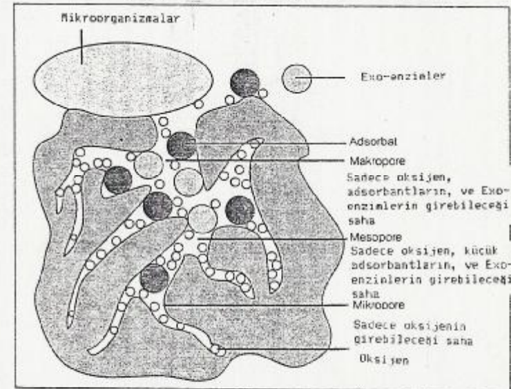
Sekil 7 : Bir biyolojik ayrışmada mikroorganizmanın yerleşmesi için kullanılan bir taşıyıcı maddenin şeması
