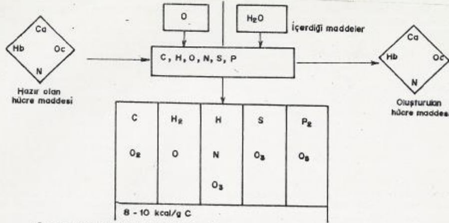
Şekil 7.1 Organik maddelerin ayrışması
