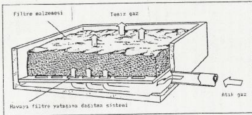
Sekil 3 : Bir biyofiltrenin alan biyofiltresi şeklinde inşaatı
