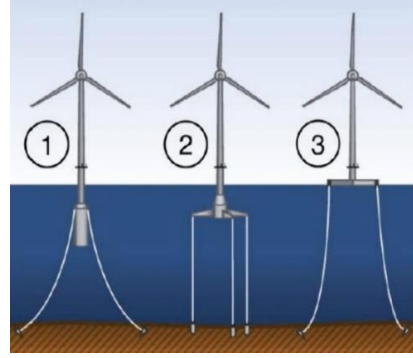
Şekil 7. Yüzer temel modelleri [43]
