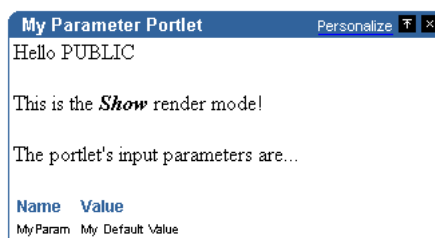
Figure 7–4 Parameter Portlet
